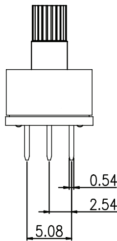
ACTUATOR
